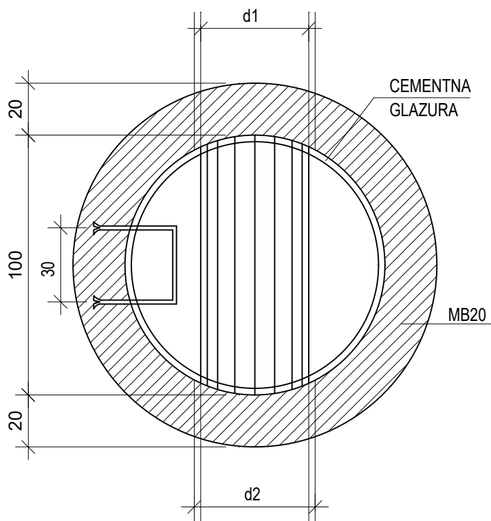
Presjek A-A
